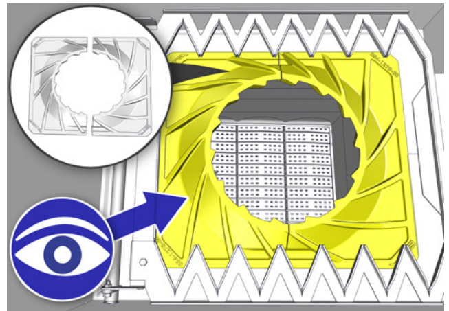
Sl. 6-10: Pokrov zgorovalne komore
