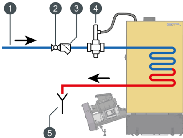
Sl. 3-3: Terminično izpustno varovalo
