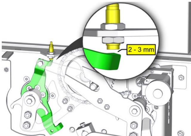
Sl. 6-22: Pravilna razdalja
