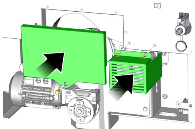
Sl. 6-20: Pokrovi
