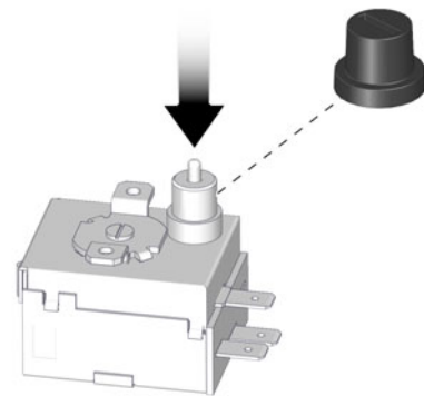
Sl. 3-4: Sprostitev varnostnega temperaturnega omejevala
