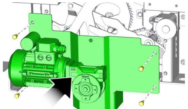
Sl. 6-19: Pogon
