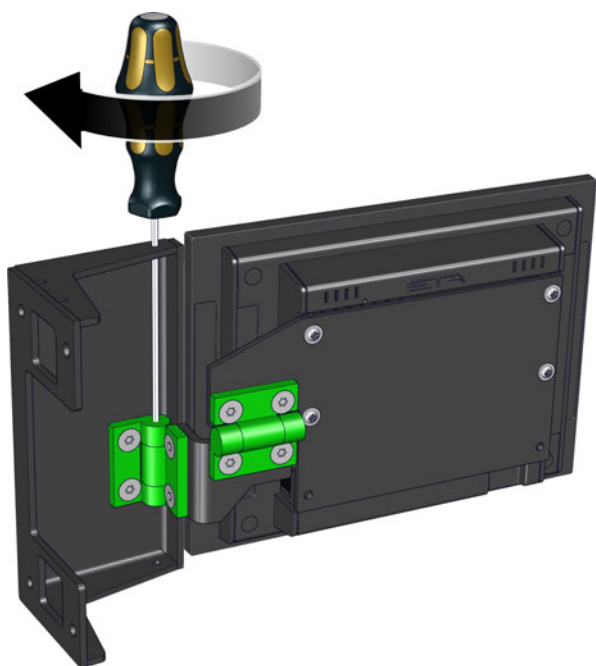
Sl. 2-5: Tečaji
