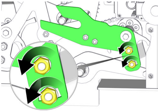
Sl. 6-15: Matici
