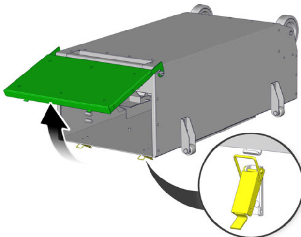
Sl. 4-3: Pokrov
