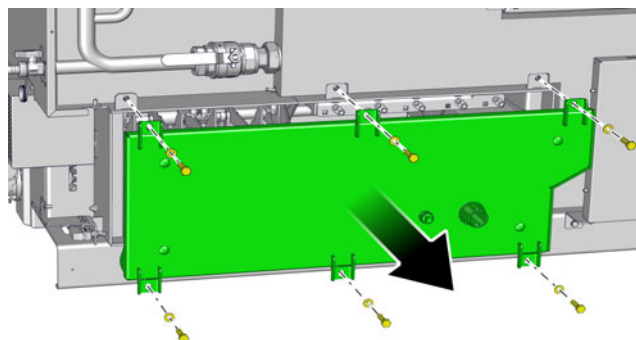
Sl. 6-23: Vzdrževalni pokrov
