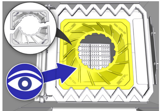
Sl. 6-10: Pokrov zgorevalne komore
