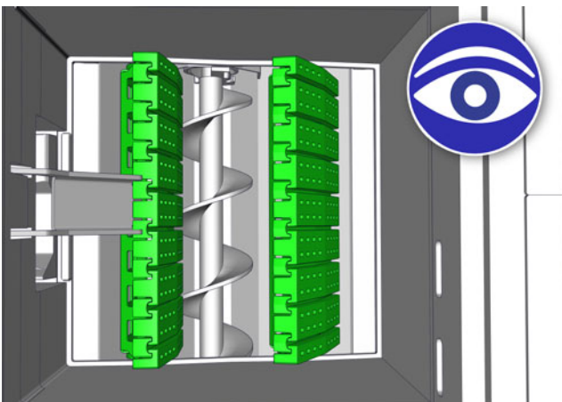
Sl. 6-9: Obrnjena nagibna rešetka
