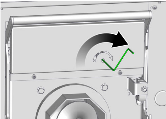
Sl. 6-8: Pravilna smer vrtenja za kotle z odvzemanjem goriva na levi strani
