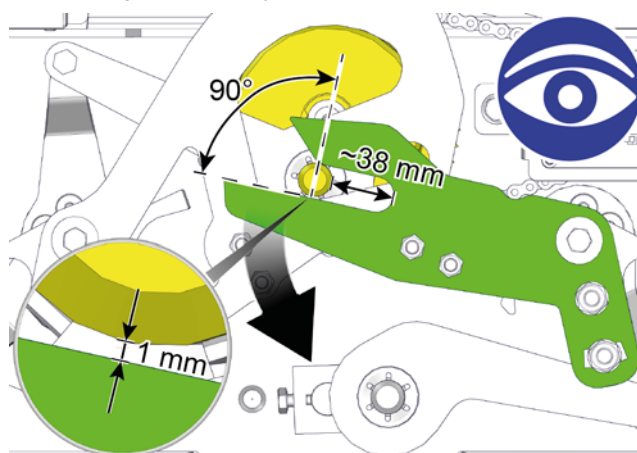
Sl. 6-14: Kontrola razdalje
