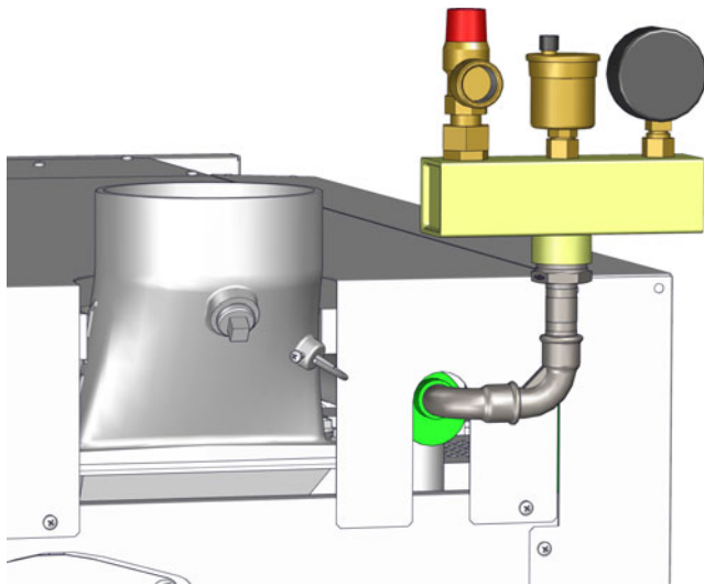
Sl. 3-6: Priključek
