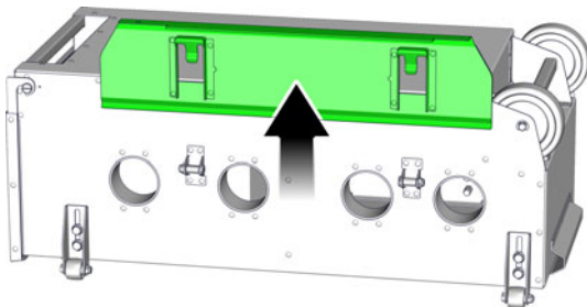
Sl. 4-7: Prekrivna pločevina
