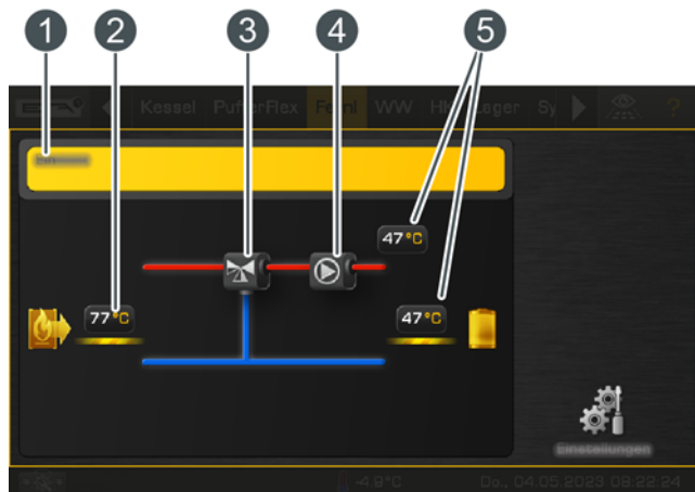
Sl. 6-118: Daljinsko ogrevanje z mešalnim ventilom
