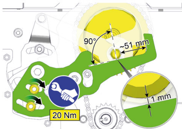
Sl. 8-18: Odzemanje na levi strani
