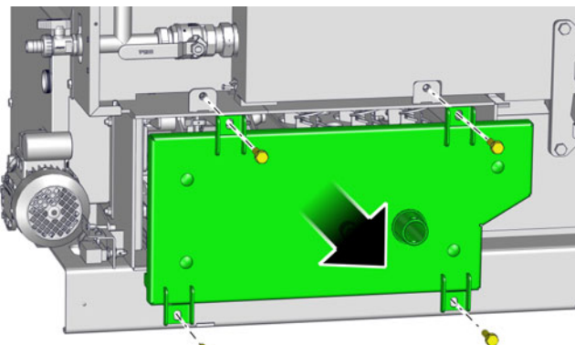
Sl. 8-22: Vzdrževalni pokrov
