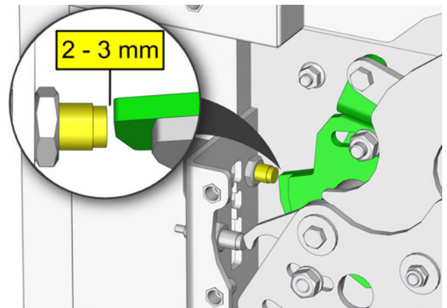
Sl. 8-25: Pravilna razdalja
