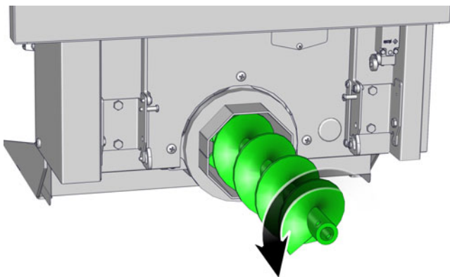
Sl. 8-5: Odvijanje polža za pepel
