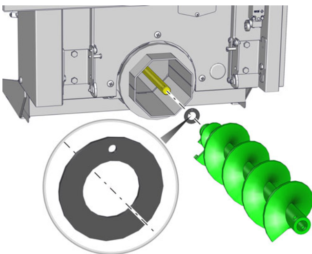
Sl. 8-6: Vstavljanje drsne podložke
