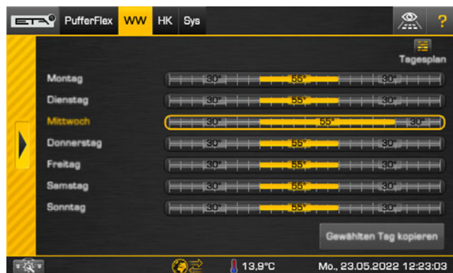
Sl. 6-29: Pregled
