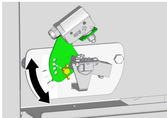
Sl. 4-3: Nastavljivo nivojsko stikalo žerjavnice
