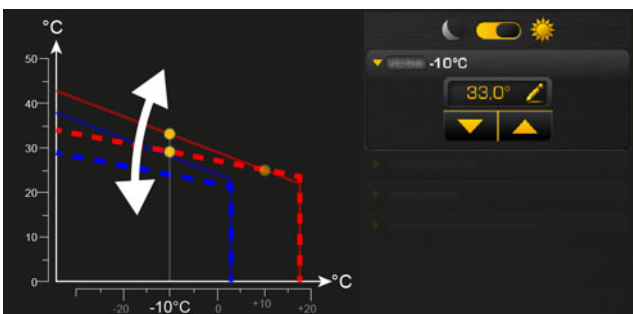
Sl. 6-101: Prilagoditev ogrevalne krivulje (pri zunanjih temperaturah pod lediščem)
