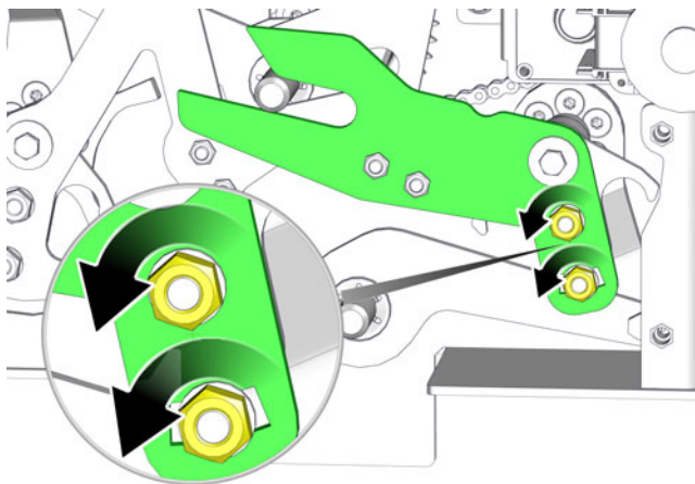
Sl. 8-16: Matici
