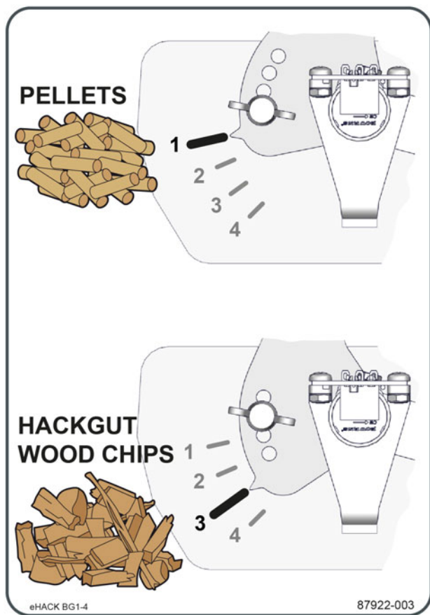
Sl. 4-4: Položaji
