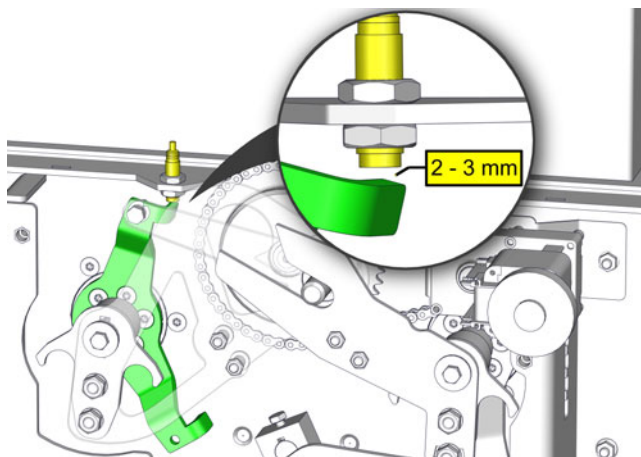
Sl. 8-23: Pravilna razdalja
