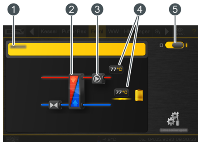
Sl. 6-119: Daljinsko ogrevanje kot predajna postaja
