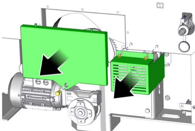
Sl. 8-22: Pokrovi
