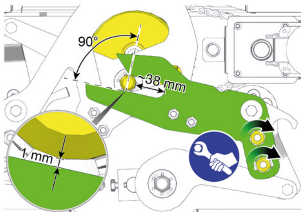
Sl. 8-17: Odvzemanje na levi strani
