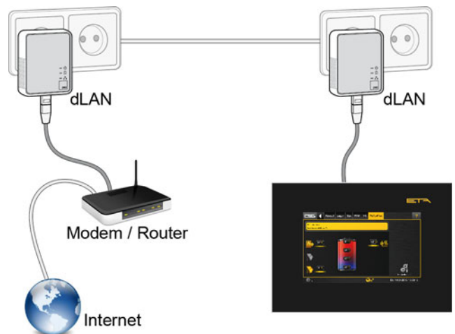
Sl. 6-33: Omrežje dLAN
