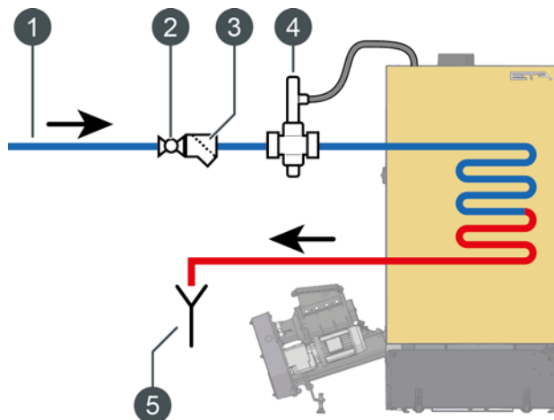
Sl. 3-3: Termično izpustno varovalo
