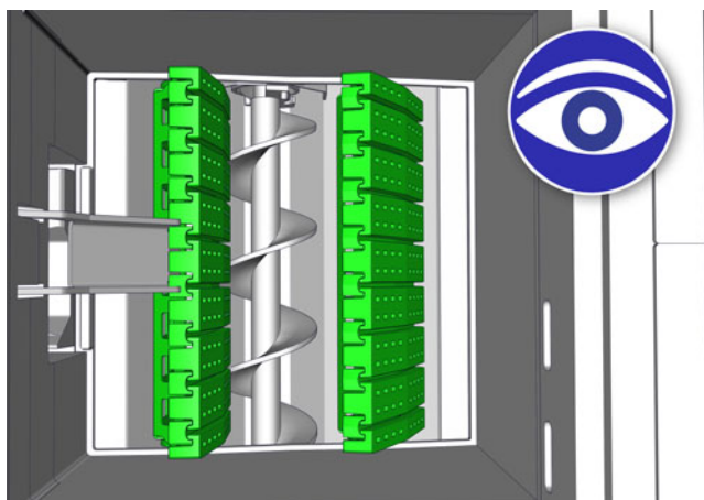
Sl. 8-10: Obrnjena nagibna rešetka
