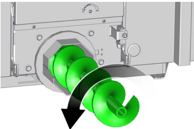
Sl. 8-5: Odvijanje polža za pepel
