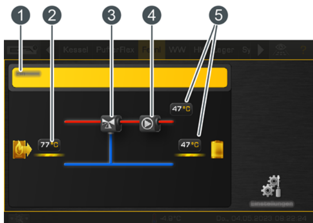
Sl. 6-118: Daljinsko ogrevanje z mešalnim ventilom
