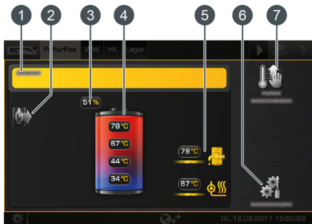
Sl. 6-78: Pregled
