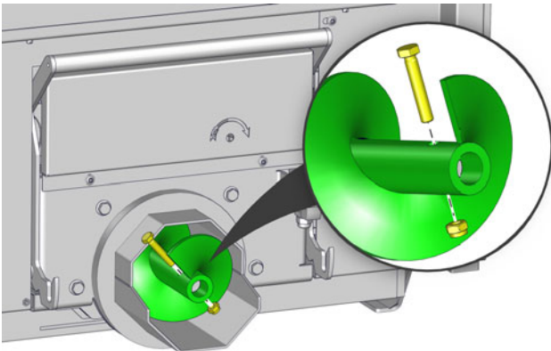
Sl. 8-4: Odstranjevanje vijaka
