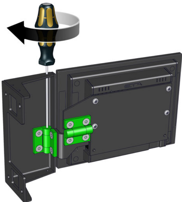
Sl. 2-5: Tečajji
