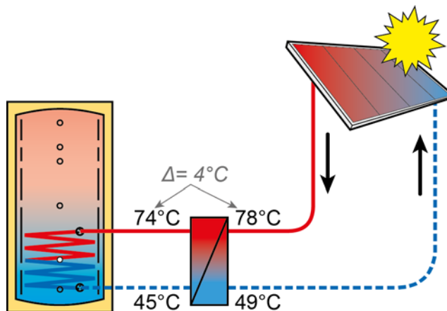
Sl. 6-109: Princip regulacije
