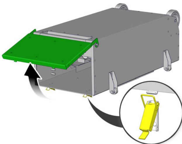
Sl. 5-3: Pokrov
