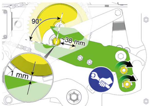
Sl. 8-18: Odvzemanje na desni strani
