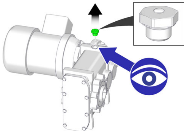
Sl. 7-11: Odzračevalni vijak
