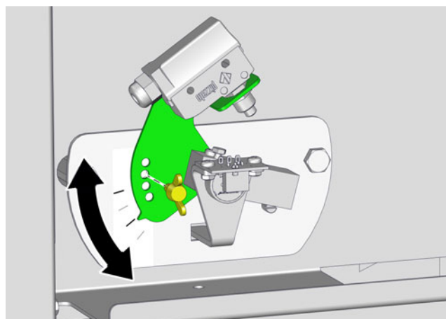
Sl. 4-3: Nastavljivo nivojsko stikalo žerjavice
