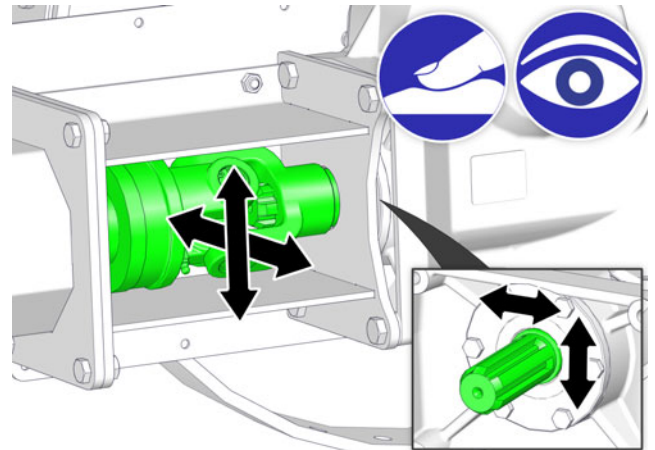
Sl. 7-3: Zračnost ležaja na vhodu v gonilo
