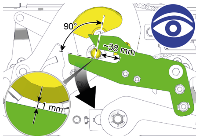
Sl. 8-15: Kontrola razdalje
