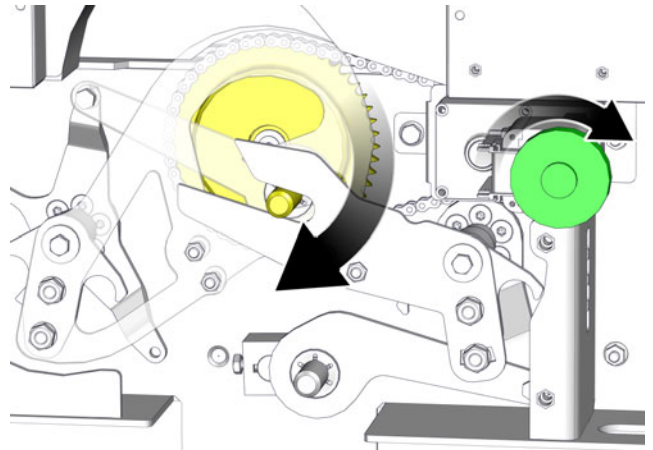
Sl. 8-14: Ročica
