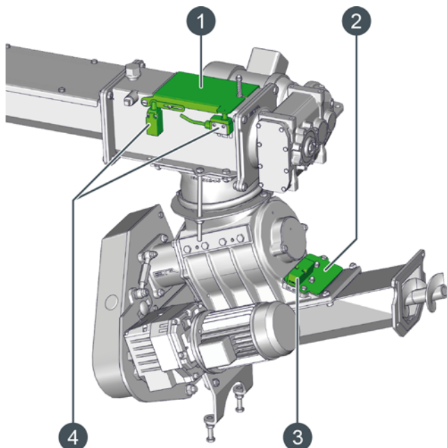
Sl. 8-1: Dostopi za odpravljanje blokad
