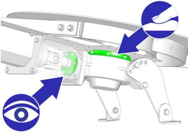
Sl. 7-1: Preverjanje uhajanja olja
