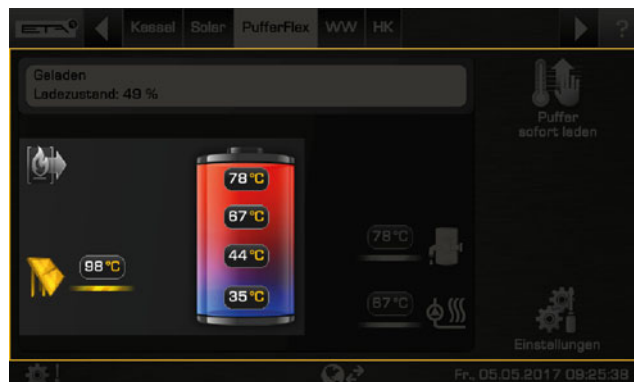
Sl. 6-82: Solarna naprava na hranilniku toplote
